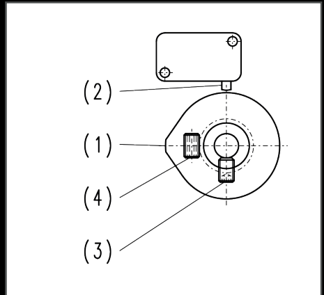
Detailansicht Endschalternocke
