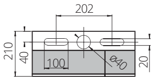
Montagewinkel links
