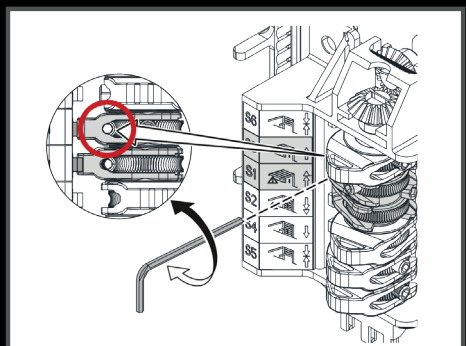
Feineinstellung Endlage
