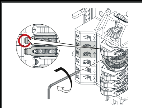
Grobeinstellung Endlage
